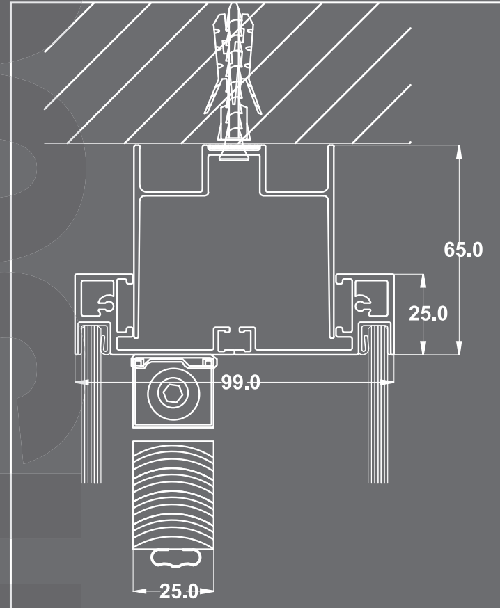
ÇİFT CAM PROFİLİ MODÜL TAVAN BİRLEŞİMİ
