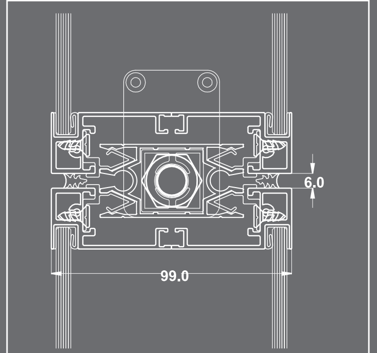
İKİ ÇİFT CAM PROFİL MODÜL BİRLEŞİMİ
