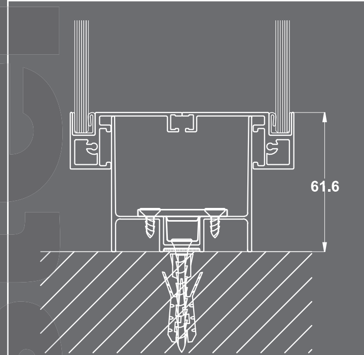
ÇİFT CAM PROFİLİ MODÜL ZEMİN BİRLEŞİMİ
